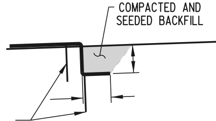
LONGITUDINAL TRENCH ANCHOR DETAIL
